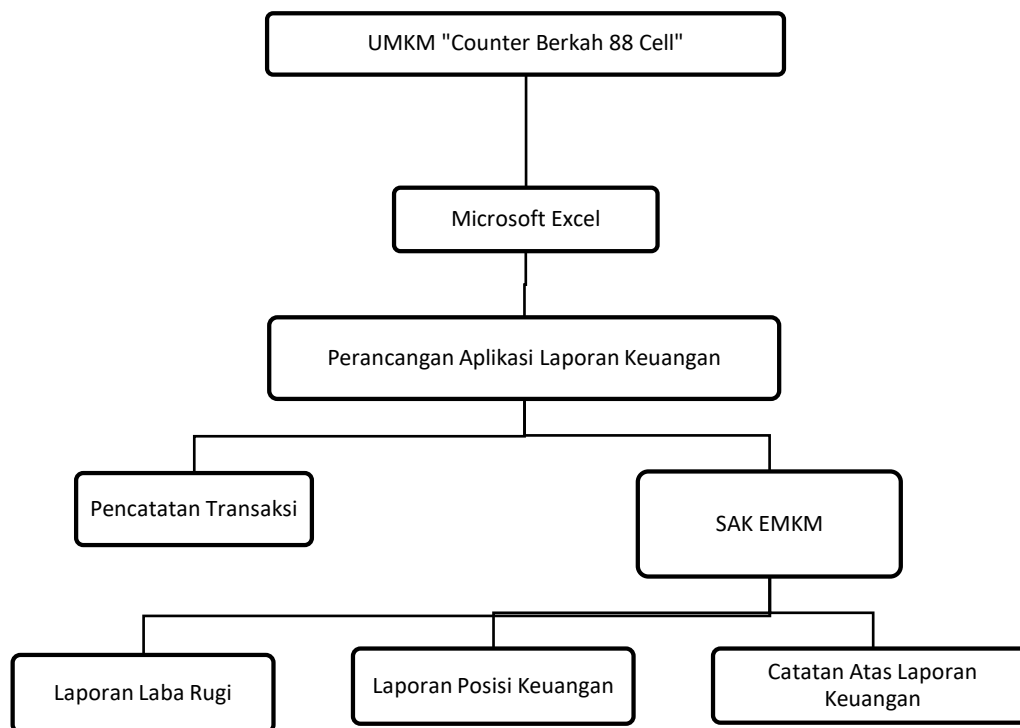
Gambar 1 Rerangka Pemikiran
